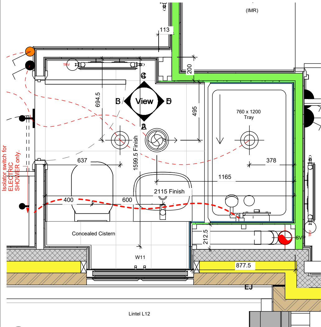
1 Ensuite Layout 1 : 20
